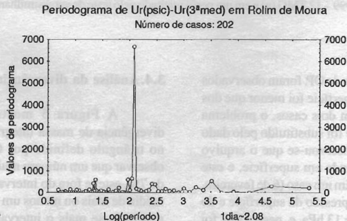
Figura 3. Periodograma da diferença de umidade relativa (%) entre o psicrômetro e a 3ª medida em Rolim de Moura-RO.
